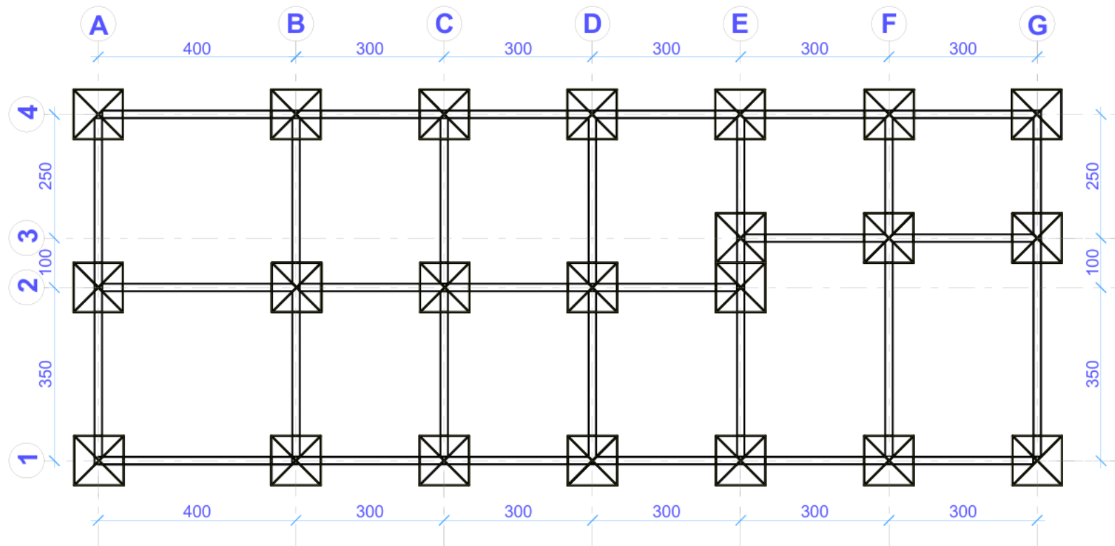
PLAN DE FONDATION
